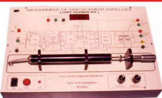
DISPLACEMENT USING LVDT
